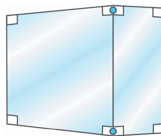
1335 Suporte de união de 2 vidros a 135 graus
