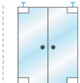
1009G Pivô superior para dobradiça 1101G
